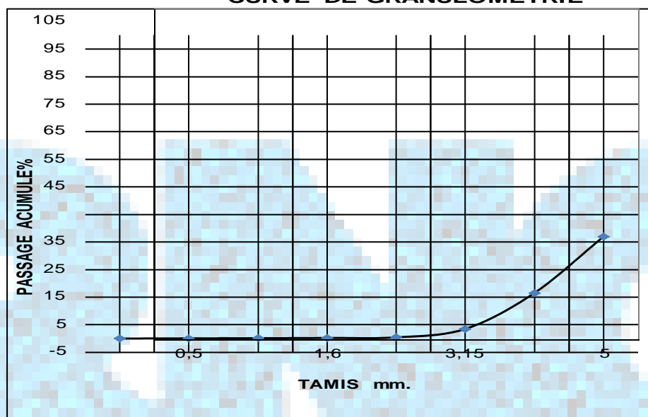
CURVE DE GRANULOMETRIE
